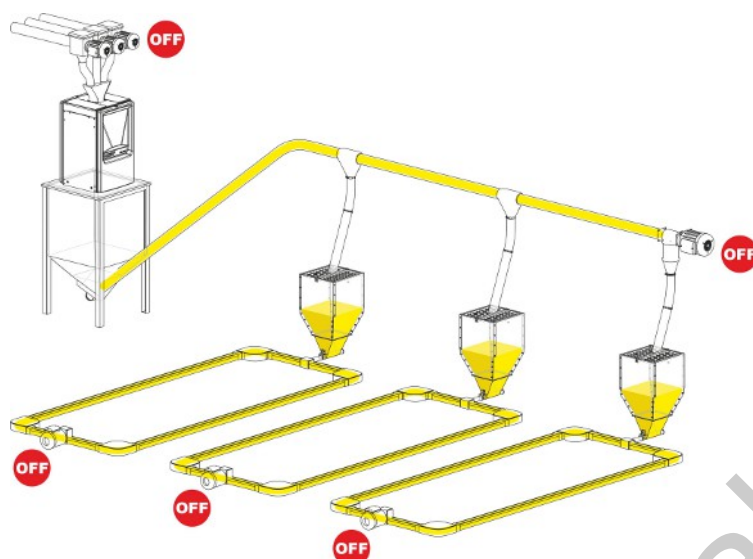
Figuur 8: De vultrechters en dwarsvijzel worden gevuld, zodat het gehele invoersysteem met invoer wordt gevuld voordat de volgende invoer begint.
