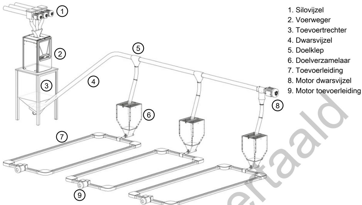
Figuur 7: In principe is het invoersysteem als volgt gestructureerd
