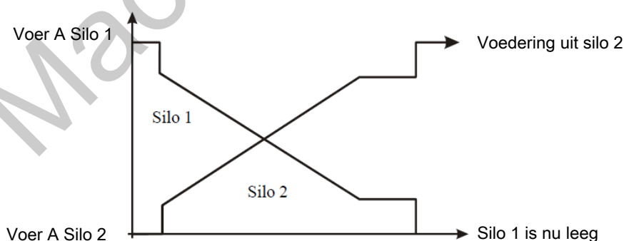
Figuur 14: Wanneer de inhoud van de silo een bepaalde hoeveelheid bereikt, begint de geleidelijke overschakeling naar een andere silo.
